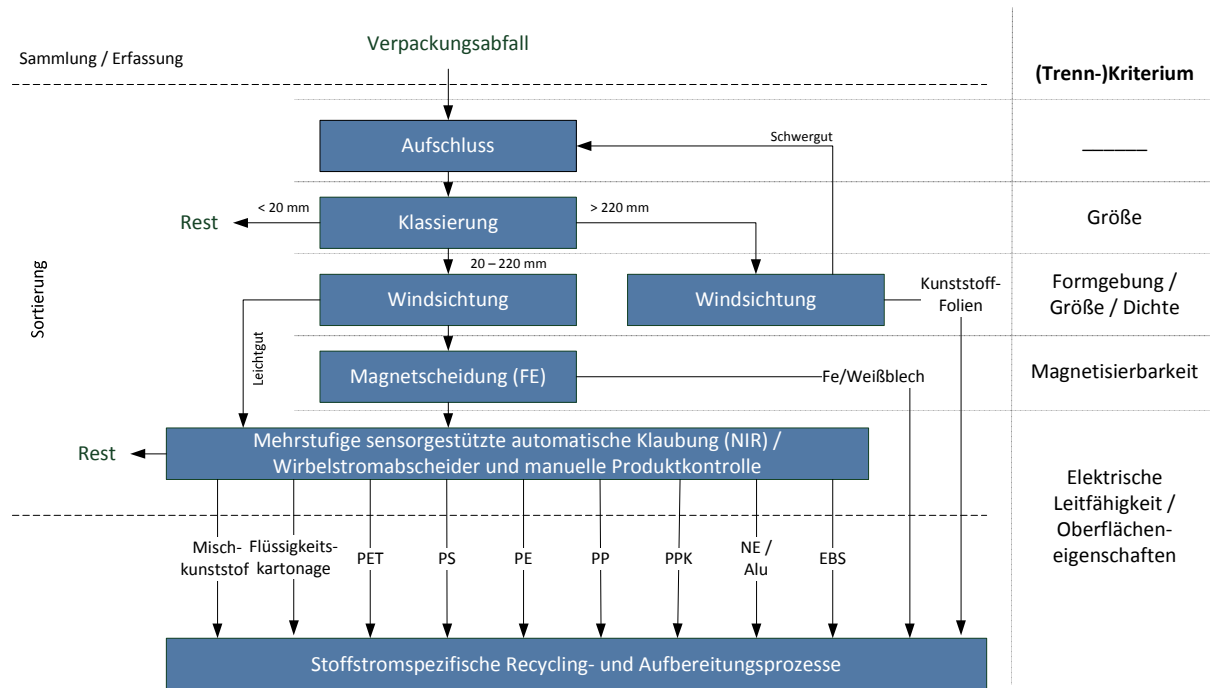
Abbildung 3-1: Prozessschritte LVP-Sortierung
