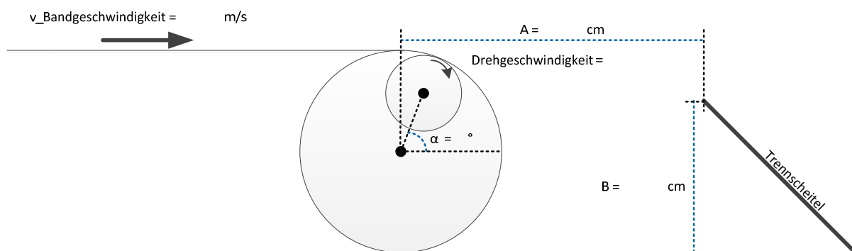
Abbildung 6.2: Skizze eines Wirbelstromscheiders mit exzentrisch gelagertem Polrad und den wichtigsten Einstellparametern (Bandgeschwindigkeit, Winkel der Poltrommel, Drehgeschwindigkeit, Abstand und Höhe Trennscheitel)
