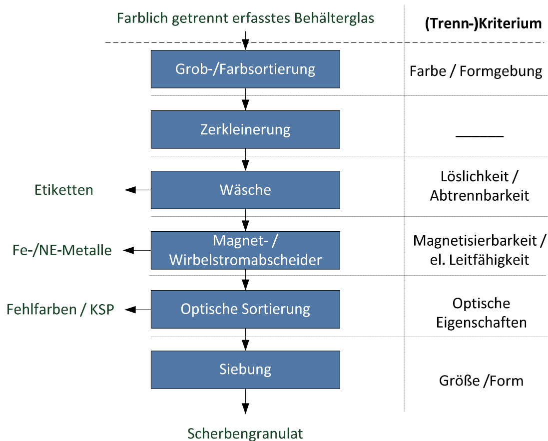
Abbildung 3-9: Prozessschritte Behälterglasrecycling
